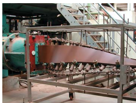
3 Poté se nepetržitě dopravuje do mixérů, kam se přidává voda, aby se vytvořil materiál s ideální konzistencí pro výrobu krytin. Všechny vzduch se odstraní, když se materiál dostává ven přes extruder.
